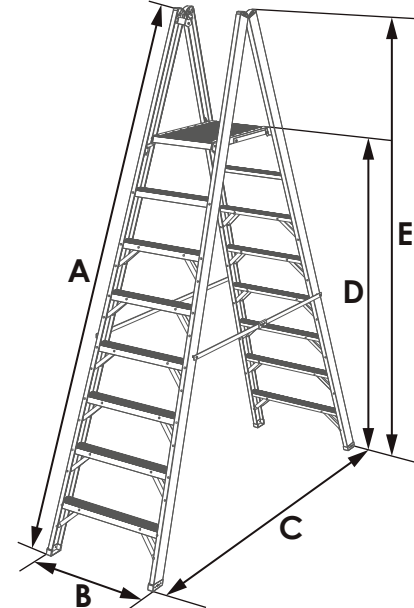
Escalera abierta
